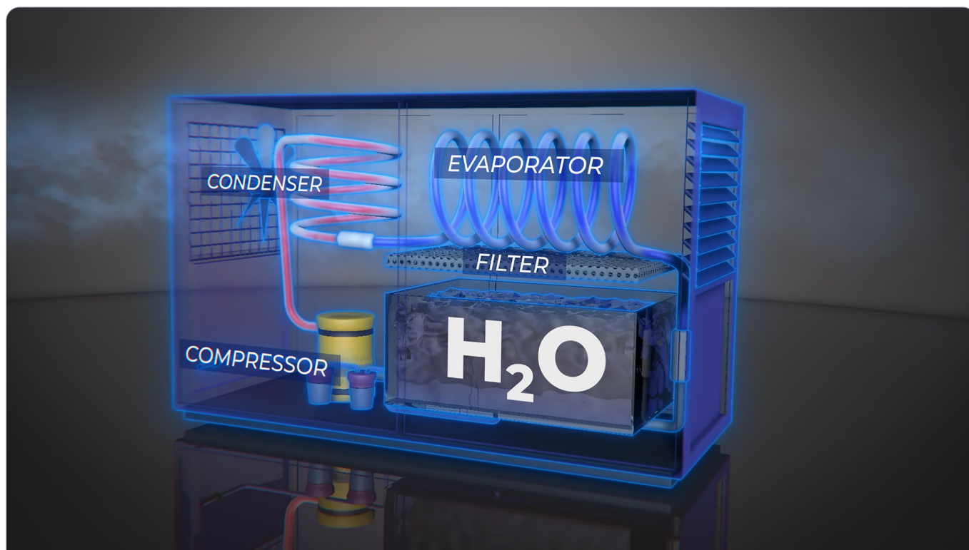
Obrázek 124 Na obrázku je schematicky znázorněn generátor atmosférické vody, ilustrující jeho součásti a princip fungování
