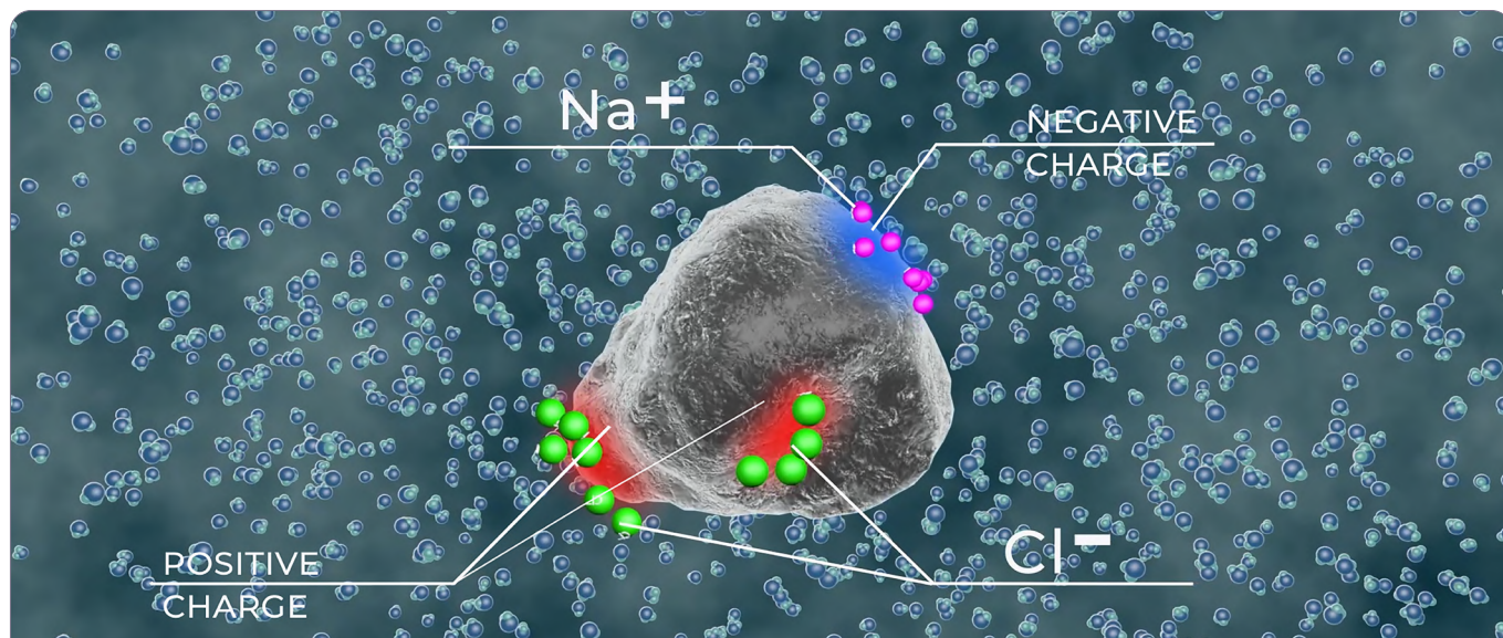
Obrázek 58 Schematické znázornění procesu tvorby hydratačního obalu kolem nabitých nanočástic plastu: v tomto procesu nanočástice díky svému náboji přitahují ionty, což napomáhá shlukování molekul vody kolem nich, a tím vytváření ochranného hydratačního obalu.
