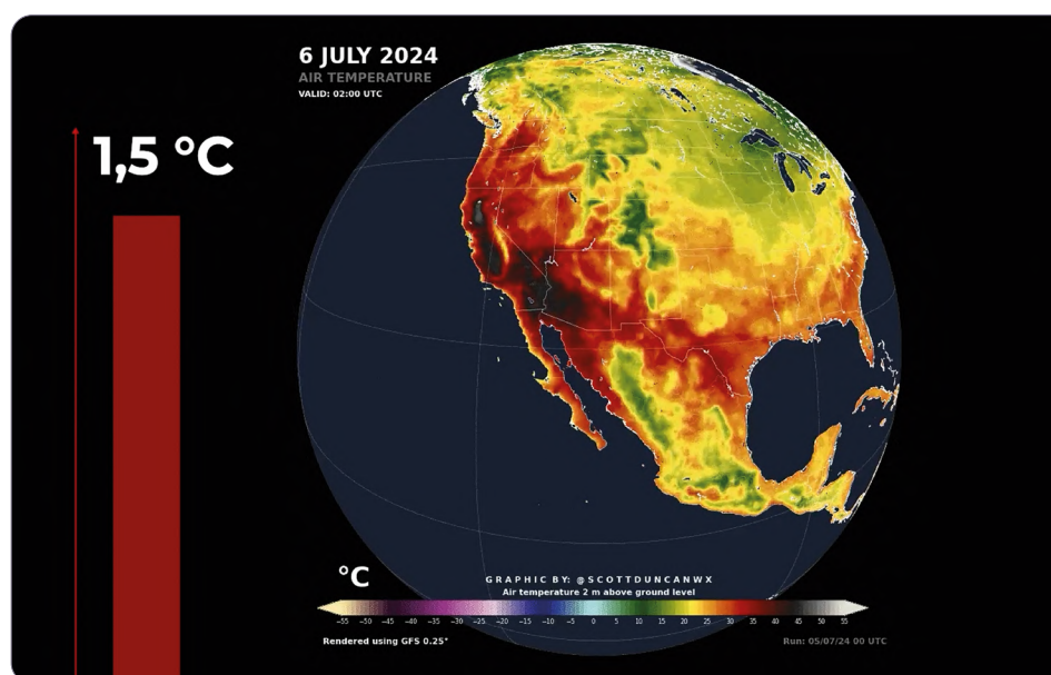
Obrázek 44 Schematické znázornění klimatického milníku: v roce 2024 průměrná globální roční teplota poprvé překročila práh 1,5\text{ °C} ve srovnání s předindustriální úrovní
