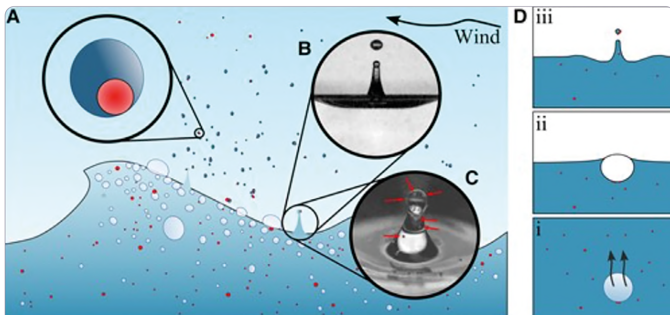
Obrázek 13 Znázornění příslušných procesů uvolňování mikroplastů z oceánu.
