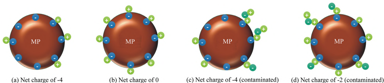
Obrázek 101 Ilustrace účinku povrchových nábojů mikroplastu způsobených znečišťujícími látkami ve vodě.
