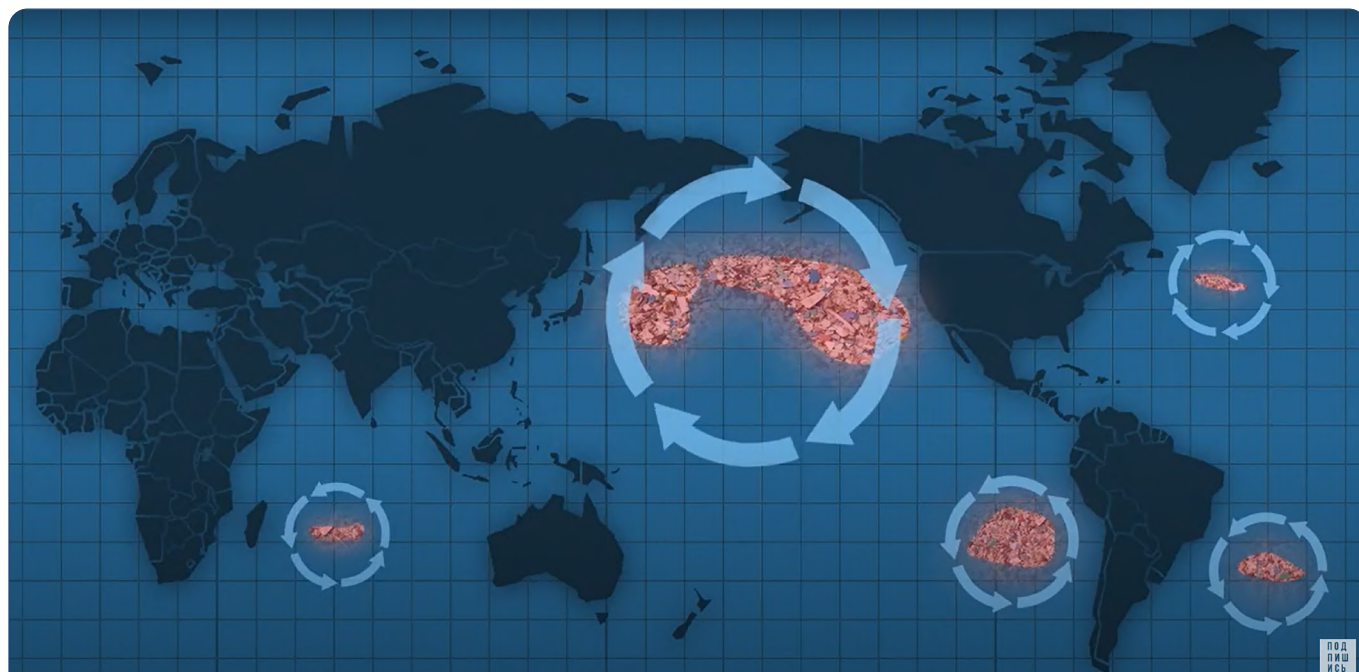
Obrázek 5 Schématické znázornění pěti velkých shromaždišť odpadu ve světovém oceánu: dvě v Atlantském oceánu, dvě v Tichém oceánu a jedno v Indickém oceánu
