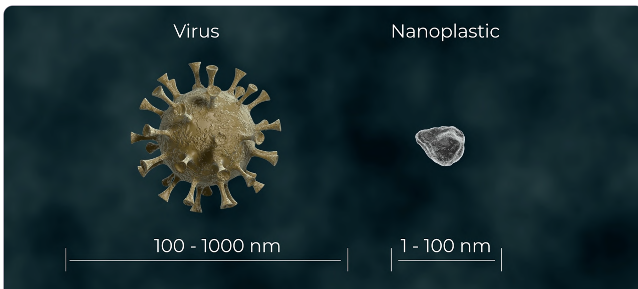
Obrázek 56 Schematické srovnání velikostí viru a částice nanoplastu.
