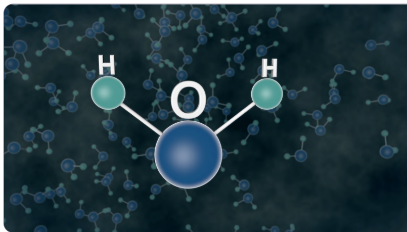
Obrázek 50 Schematické znázornění molekuly vody: dva atomy vodíku (H) jsou spojeny s jedním atomem kyslíku (O) v úhlu přibližně 104,5°, čímž vzniká dipól s kladným a záporným nábojem
