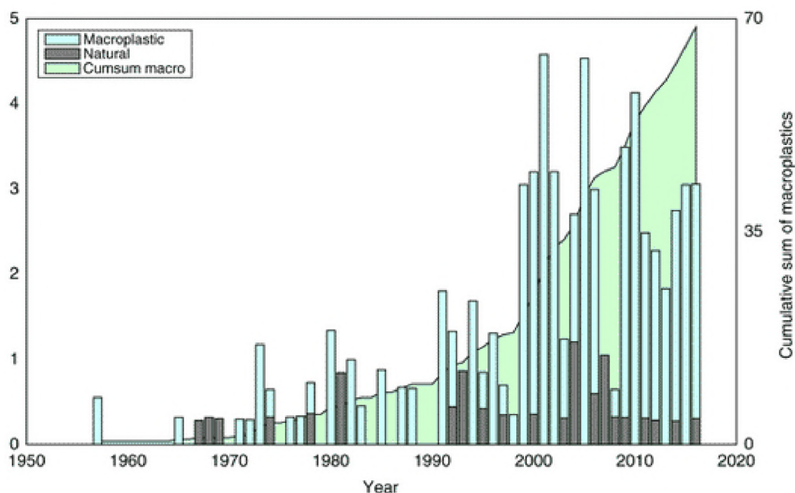
Obrázek 48 Graf nárůstu koncentrace plastů v oceánech za poslední desetiletí. Kumulativní součet makroplastů zachycených v oceánu a údaje pro jednotlivé roky.
