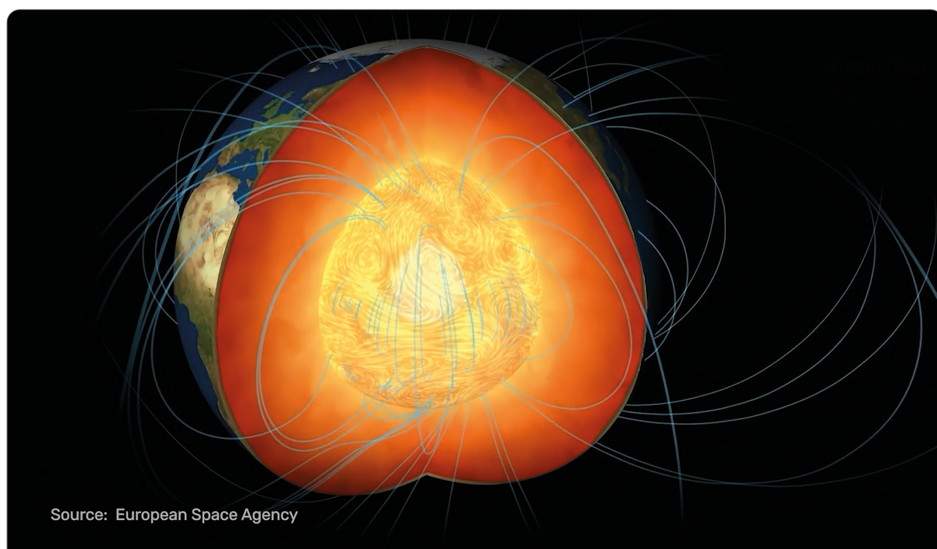
Obrázek 65 Schematické znázornění procesu vzniku geomagnetického pole: kapalné vnější jádro Země se otáčí kolem pevného vnitřního jádra a vytváří přirozený generátor – geodynamo, díky němuž vzniká magnetické pole planety.
