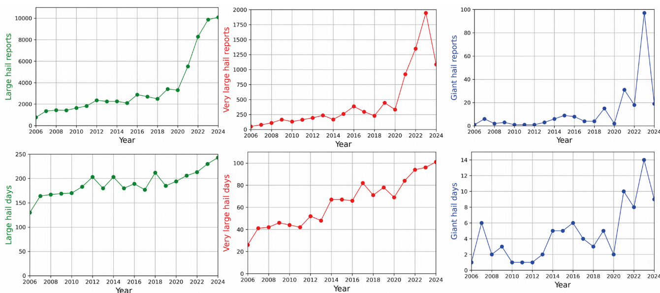
Obrázek 63 Počet hlášení a dní s velkými (2+ cm), velmi velkými (5+ cm) a obrovskými (10+ cm) kroupami v období od roku 2006 do roku 2024.
