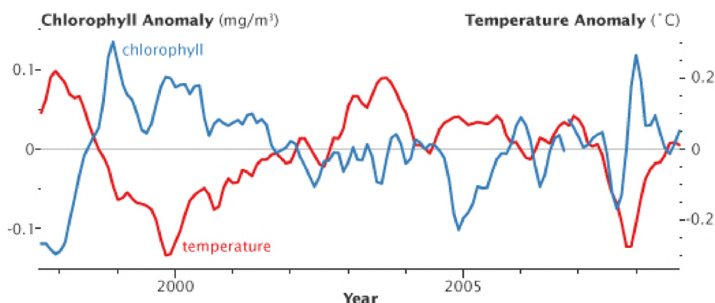
Obrázek 41 Přibližně 70 % oceánu je trvale rozčleněno do vrstev, které se mezi sebou špatně mísí. V období od konce roku 1997 do poloviny roku 2008 satelity zaznamenávaly, že teploty vyšší než průměrné (červená linie) vedly v těchto oblastech ke koncentraci chlorofylu nižší než průměrné (modrá linie). (Graf upraven podle Behrenfeld et al. 2009, Robert Simmon)
