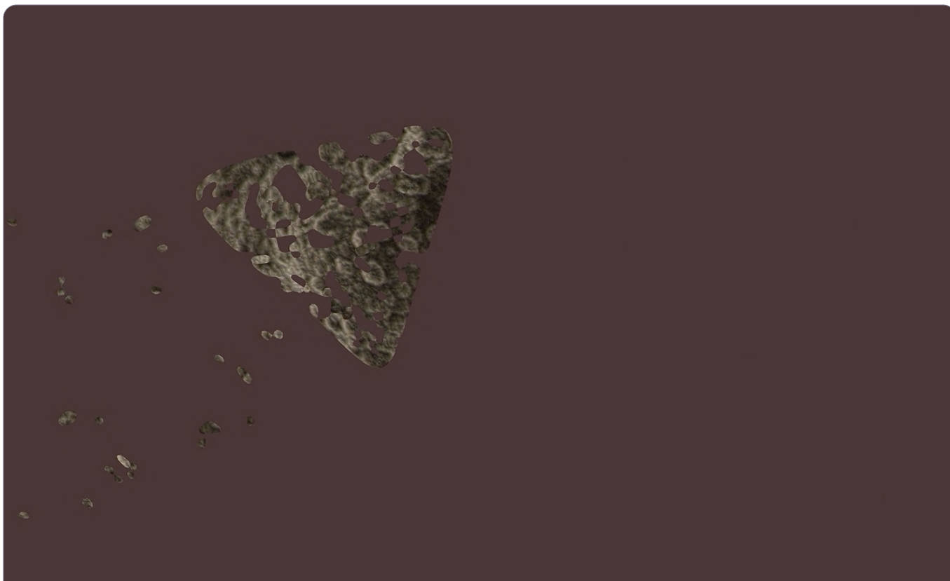
Obrázek 6 Schematické znázornění procesu fragmentace plastových částic až na nanoúroveň při zachování polymerní struktury
