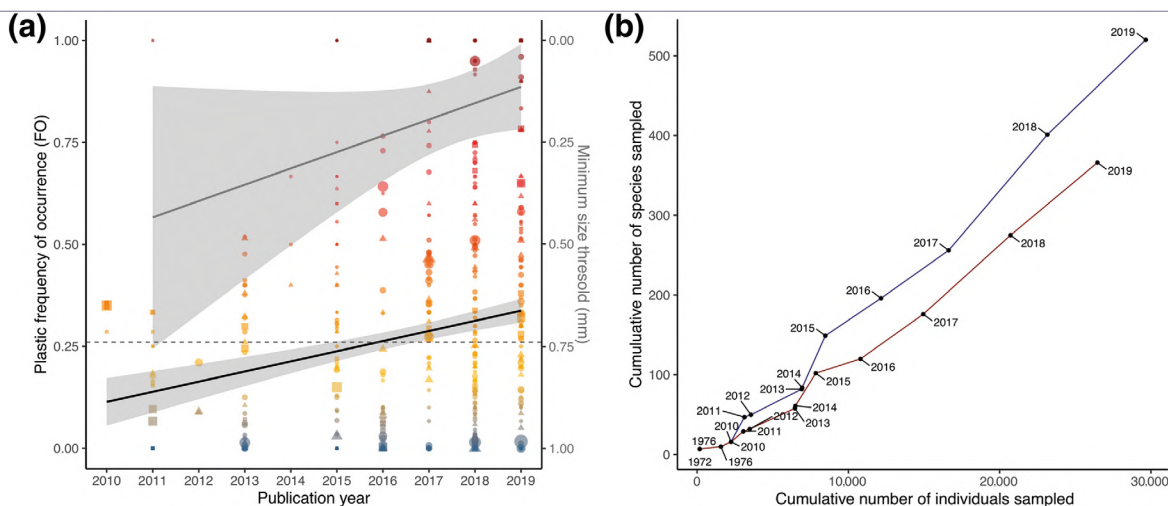
Obrázek 30 Časové trendy spotřeby plastů rybami (a) Horní šedá čára ukazuje, že od roku 2011 je patrný trend objevování stále menších částic. Dolní černá čára znázorňuje nárůst frekvence výskytu plastů (FO) u všech druhů ryb v období od roku 2010 do 2019. V tomto období spotřeba plastů významně rostla tempem 2,4 % ročně. Vodorovná tečkovaná čára představuje FO 0,26 – průměrnou frekvenci spotřeby plastů rybami na celém světě. (b) Křivka akumulace druhů, kde modrá čára označuje kumulativní počet druhů zkoumaných v průběhu času, včetně druhů, u kterých byl plast zjištěn i nezjištěn, a červená čára znázorňuje pouze druhy s prokázaným požitím plastu. Absence asymptoty na červené křivce ukazuje na vysokou pravděpodobnost, že se v následujících letech objeví další druhy, které budou plast požírat.
