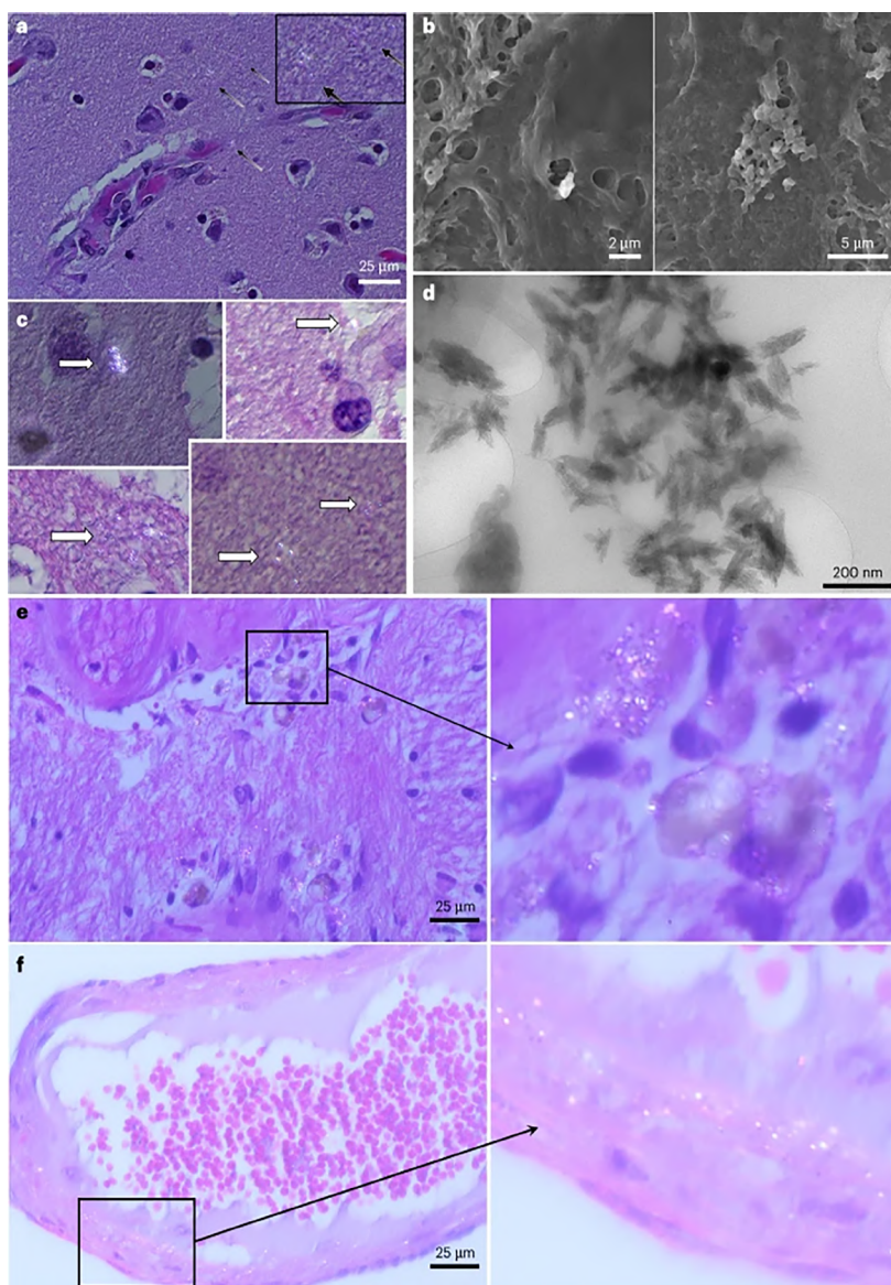
Obrázek 91 Polarizační vlnová mikroskopie (a, černé šipky označují refrakterní inkluze; vložka je digitální zvětšení pro větší přehlednost) a SEM (b, zorné pole má šířku 15,4 a 20,1 \mu\text{m} ) byly použity ke skenování řezů mozku ze vzorků zesnulých lidí. c, Velké ( >1 \mu\text{m} ) inkluze nebyly pozorovány; další příklady polarizačních vln jsou zvýrazněny (bílé šipky zvýrazňují submikronové refrakterní inkluze). Omezení rozlišení těchto technologií vedlo k použití TEM k vyšetření extraktů z pelet použitých pro Py-GC/MS. d, Příklad TEM snímků, které po disperzi dokáží rozlišit nespočet pevných částic ve formě úlomků nebo vloček, jejichž rozměry byly převážně <200 \text{ nm} na délku a <40 \text{ nm} na šířku. e, f, Polarizační vlnová mikroskopie odhalila podstatně více refrakterní inkluzí v případech demence, zejména v oblastech s akumulací imunitních buněk (e) a podél cévních stěn (f). Všechny snímky byly pořízeny u malé podskupiny účastníků ( n = 10 u normálních mozků; n = 3 u případů demence), aby poskytly vizuální důkazy na podporu analytické chemie.
