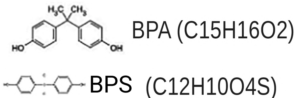
Obrázek 76 Molekulární struktury a chemické vzorce bisfenolu A (BPA) a bisfenolu S (BPS)
