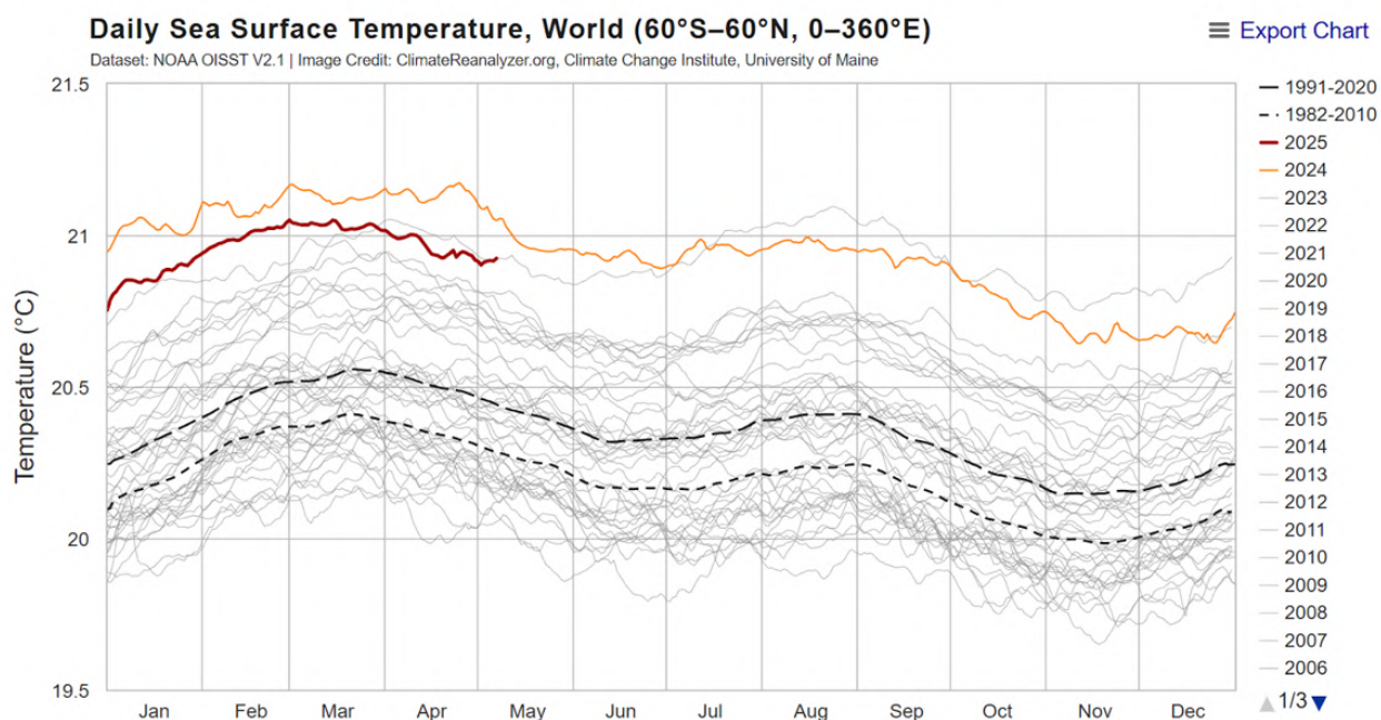
Obrázek 128 Průměrná denní teplota povrchu oceánu, 1981–2025.
