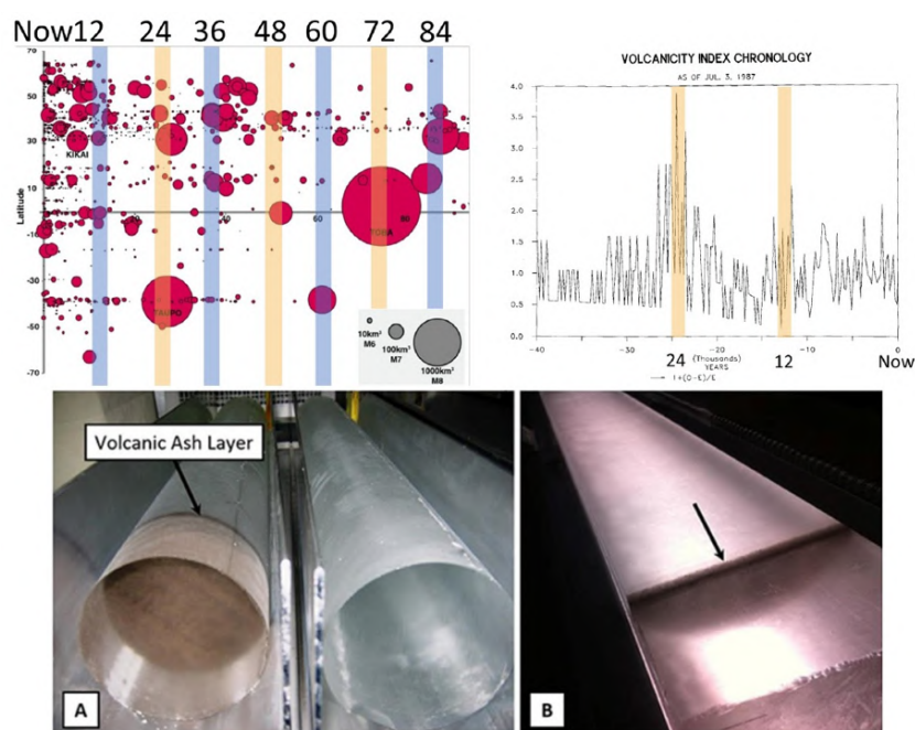
Obrázek 139 Grafy ilustrují katastrofickou vulkanickou aktivitu, k níž dochází každých 12 000 let a ještě intenzivnější události každých 24 000 let.
