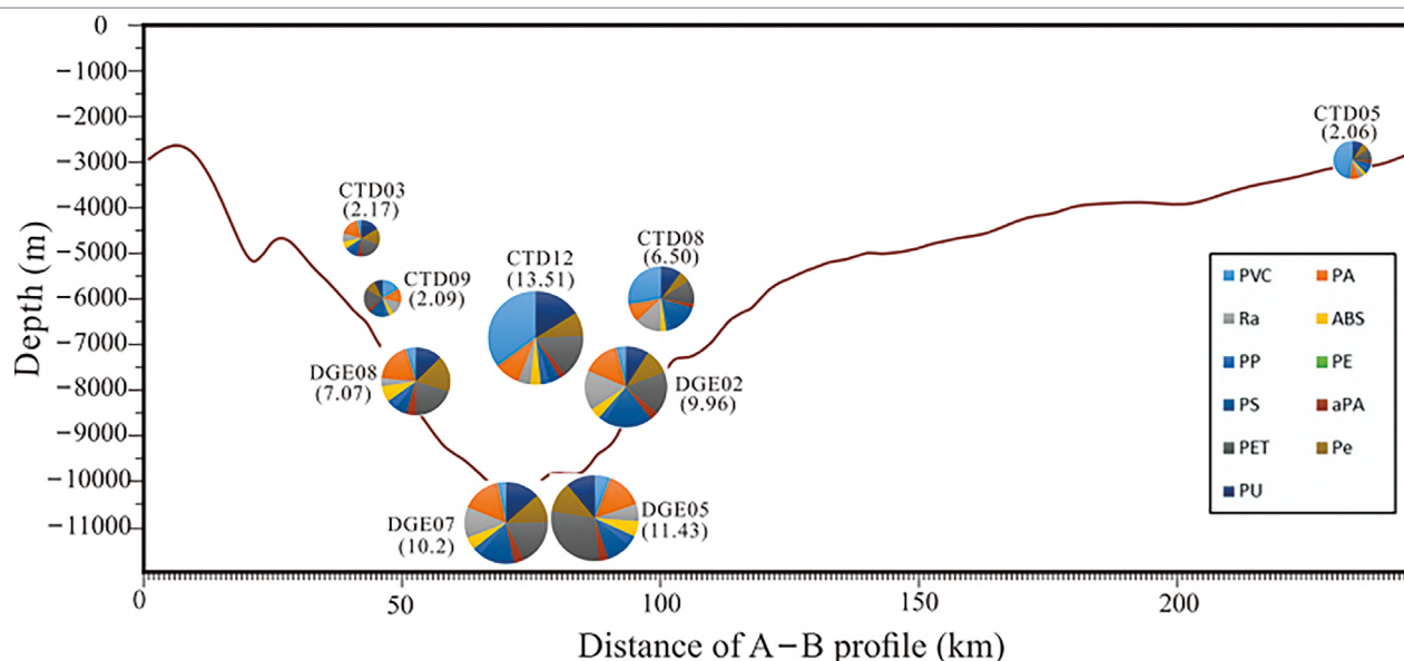
Obrázek 8 Profil rozšíření a složení mikroplastů ve vzorcích vody z Mariánského příkopu. Koláčové grafy znázorňují složení mikroplastů a čísla v závorkách udávají jejich výskyt v jednotkách kusů na liter. PVC (polyvinylchlorid), PA (polyamid), Ra (viskóza), ABS (akrylonitrilbutadienstyren), PP (polypropylen), PE (polyetylen), PS (polystyren), APA (aromatický polyamid), PET (polyethylentereftalát), PES (polyester), PU (polyuretan). Osa X odpovídá příčné linii od bodu A (12° s. š., 142,5° v. d.) do bodu B (9,8° s. š., 141,43° v. d.).
