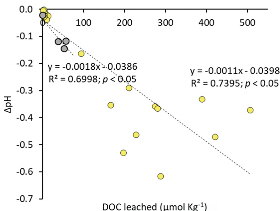
Obrázek 35 Vztahy mezi změnou pH a rozpuštěným organickým uhlíkem (DOC) vyluhovaným z plastu jsou znázorněny v grafu pro každý jednotlivý opakovaný vzorek ze všech experimentů. Zahrnuty jsou také kontrolní vzorky bez plastu pro každý experiment. Žluté body odpovídají ozařovaným vzorkům, šedé body vzorkům uchovávaným ve tmě.
