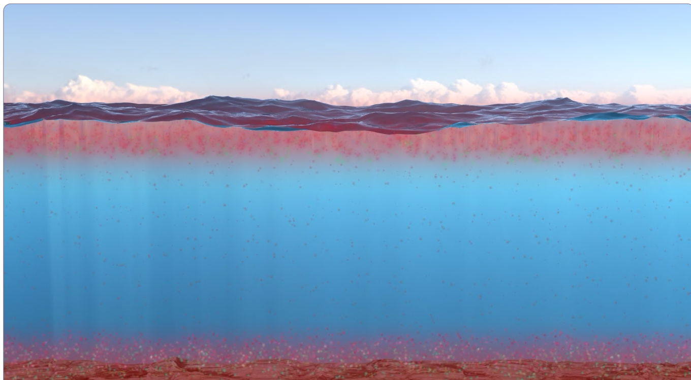
Obrázek 11 Schematické znázornění povrchové a spodní vrstvy znečištění mikro- a nanoplasty
