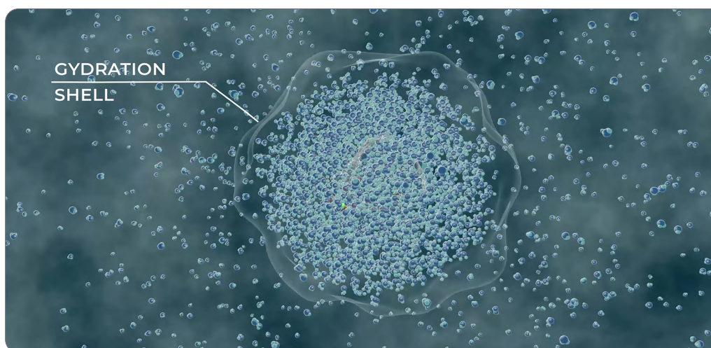
Obrázek 59 Schematické znázornění hydratačního obalu kolem částice nanoplastu
