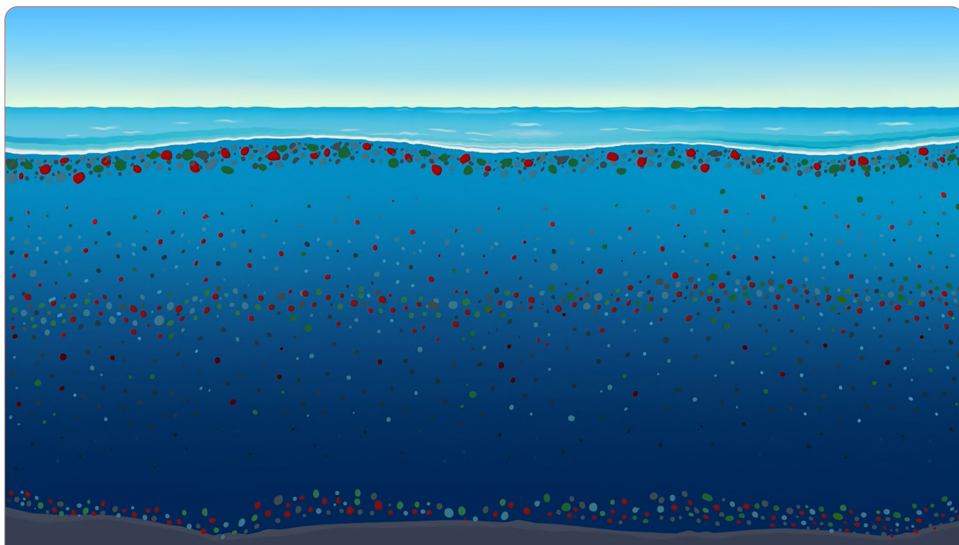
Obrázek 12 Schematické znázornění rozložení mikro- a nanoplastů v povrchové vrstvě, spodní vrstvě a v oblasti termokliny
