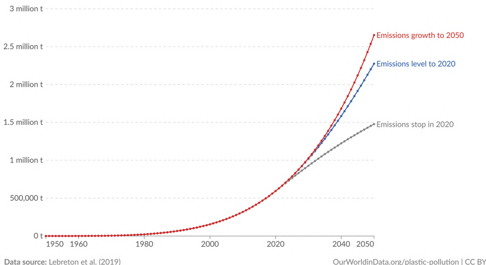
Obrázek 29 Graf nárůstu množství mikroplastů na hladině oceánu s prognózou do roku 2050.
