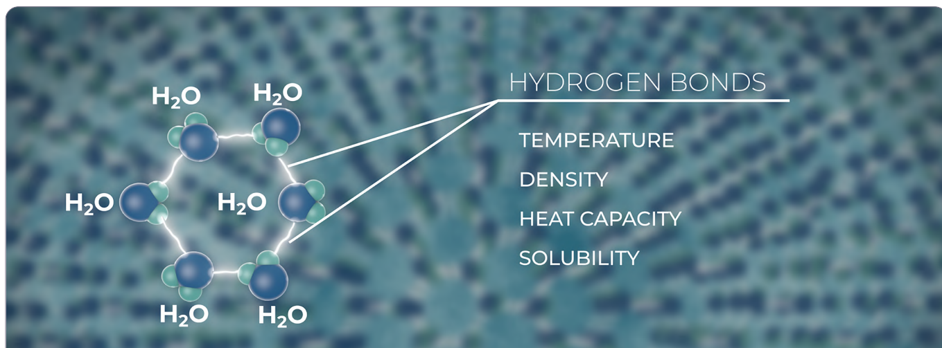
Obrázek 55 Schematické znázornění vodíkových vazeb v molekulách vody a jejich vlivu na klíčové vlastnosti vody: vodíkové vazby přispívají k vysoké měrné tepelné kapacitě vody, což jí umožňuje efektivně pohlcovat a uchovávat teplo. Tyto vazby rovněž určují hustotu vody, která je nejvyšší při 4 °C, a její schopnost rozpouštět polární a iontové látky, díky čemuž je voda univerzálním rozpouštědlem.
