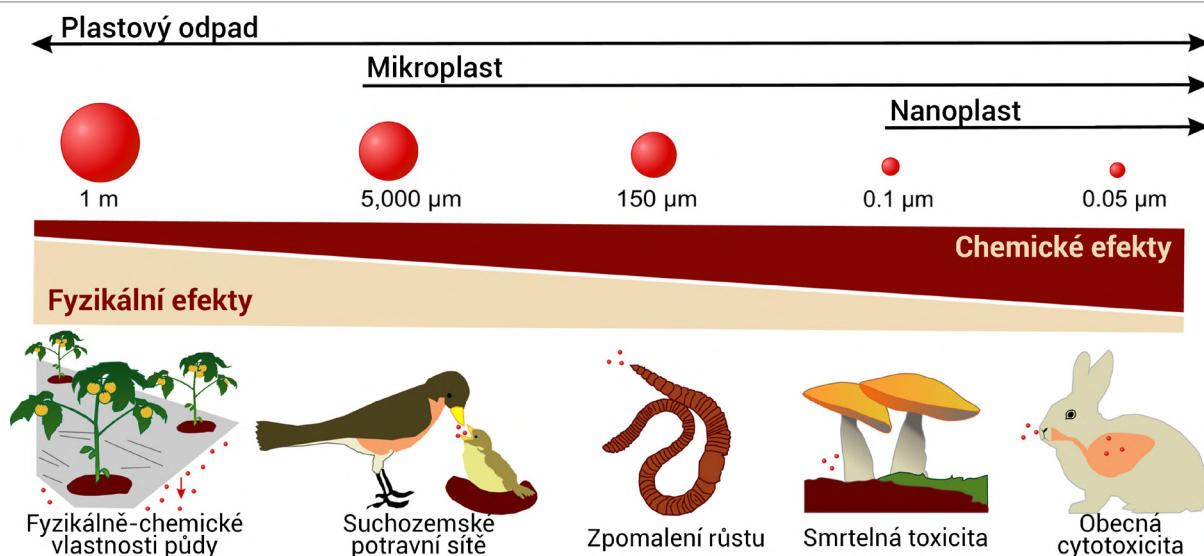
Obrázek 15 Mikroplasty jako spouštěč kombinovaných fyzikálních a chemických jevů.
