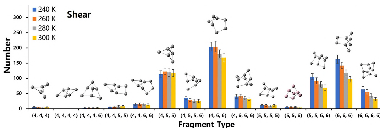
Obrázek 53 Rozložení fragmentů (struktury 3. úrovně) při různých teplotách. Všimněte si, že (4, 4, 4) označuje symbol fragmentu, který je složen ze tří čtyřčlenných kruhů.
