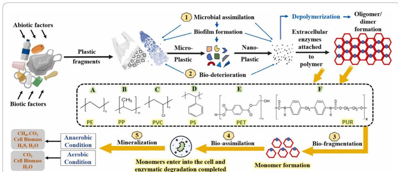
Obrázek 125 Rozklad mikro- a nanoplastů bakteriálními enzymy.
