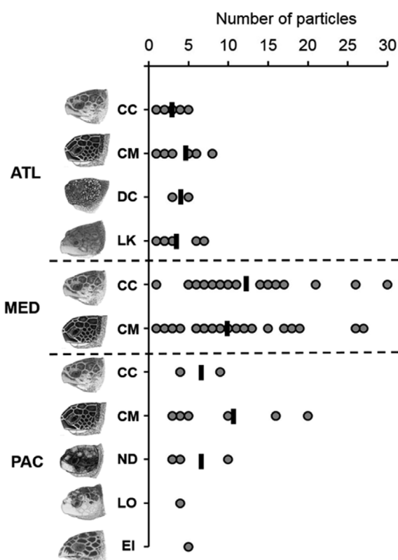
Obrázek 27 Požití syntetických mikročástic všemi druhy mořských želv ze tří oceánských pánví. Celkový počet částic identifikovaných v každém dílčím vzorku o objemu 100 ml pro každý druh v každé oceánské pánvi. Černá čára označuje průměrný počet částic. Siluety lebek mořských želv použity se souhlasem WIDECAST; původní kresby Tom McFarland.
