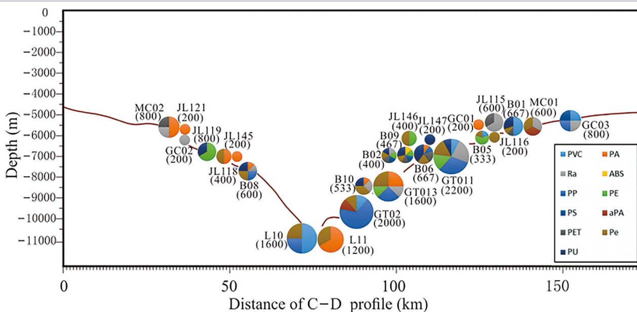
Obrázek 9 Profil rozšíření a složení mikroplastů ve vzorcích sedimentů z Mariánského příkopu. Koláčové grafy znázorňují složení mikroplastů a čísla v závorkách udávají jejich výskyt v jednotkách kusů na liter. PVC (polyvinylchlorid), PA (polyamid), Ra (viskóza), ABS (akrylonitrilbutadienstyren), PP (polypropylen), PE (polyetylen), PS (polystyren), APA (aromatický polyamid), PET (polyethylentereftalát), PES (polyester), PU (polyuretan). Osa X odpovídá příčné linii od bodu C (12° s. š., 141,9° v. d.) do bodu D (10,5° s. š., 141,3° v. d.).
