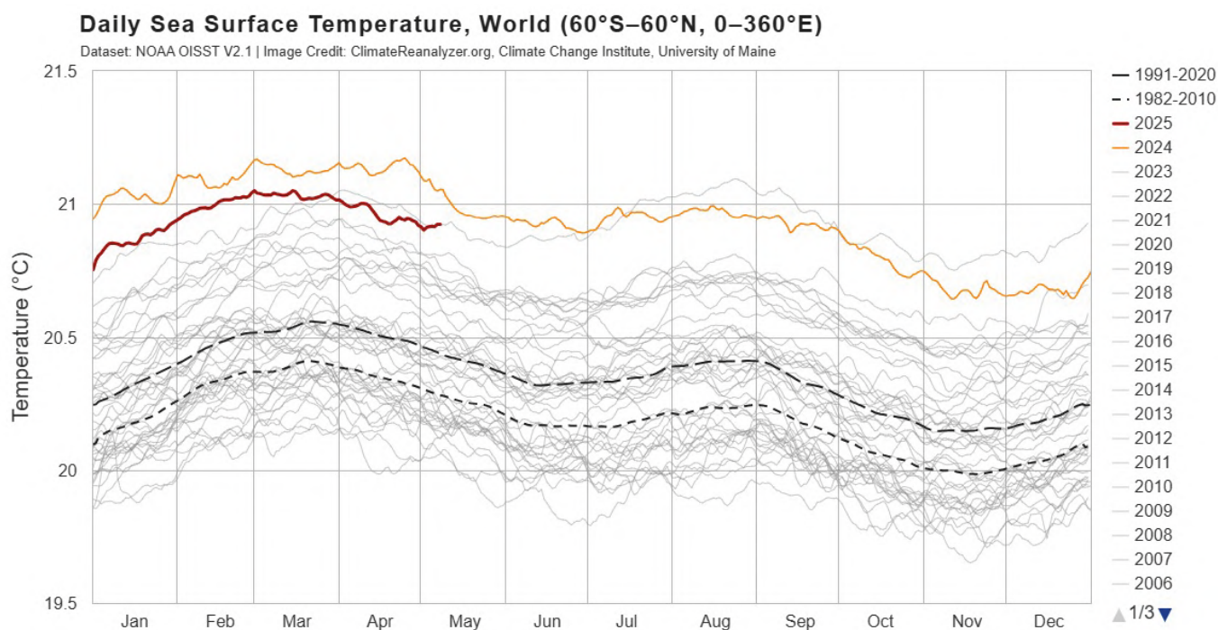
Obrázek 43 Denní hodnoty teploty mořské hladiny: grafické zobrazení změn teploty svrchní vrstvy oceánu, odrážející sezónní výkyvy v jednotlivých letech.
